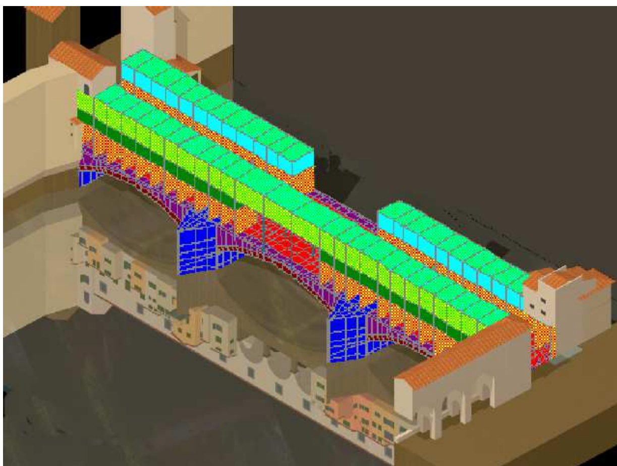
Studio delle strutture di Ponte Vecchio tramite modello agli elementi finiti in analisi non lineare.
